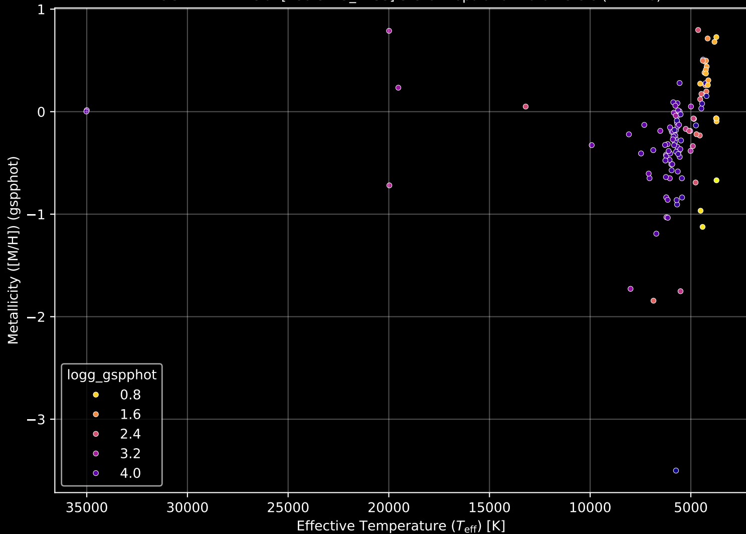
APOGEE DR17 Field: [280-32-O_TESS] Stellar Population Parameters (n= 116)
