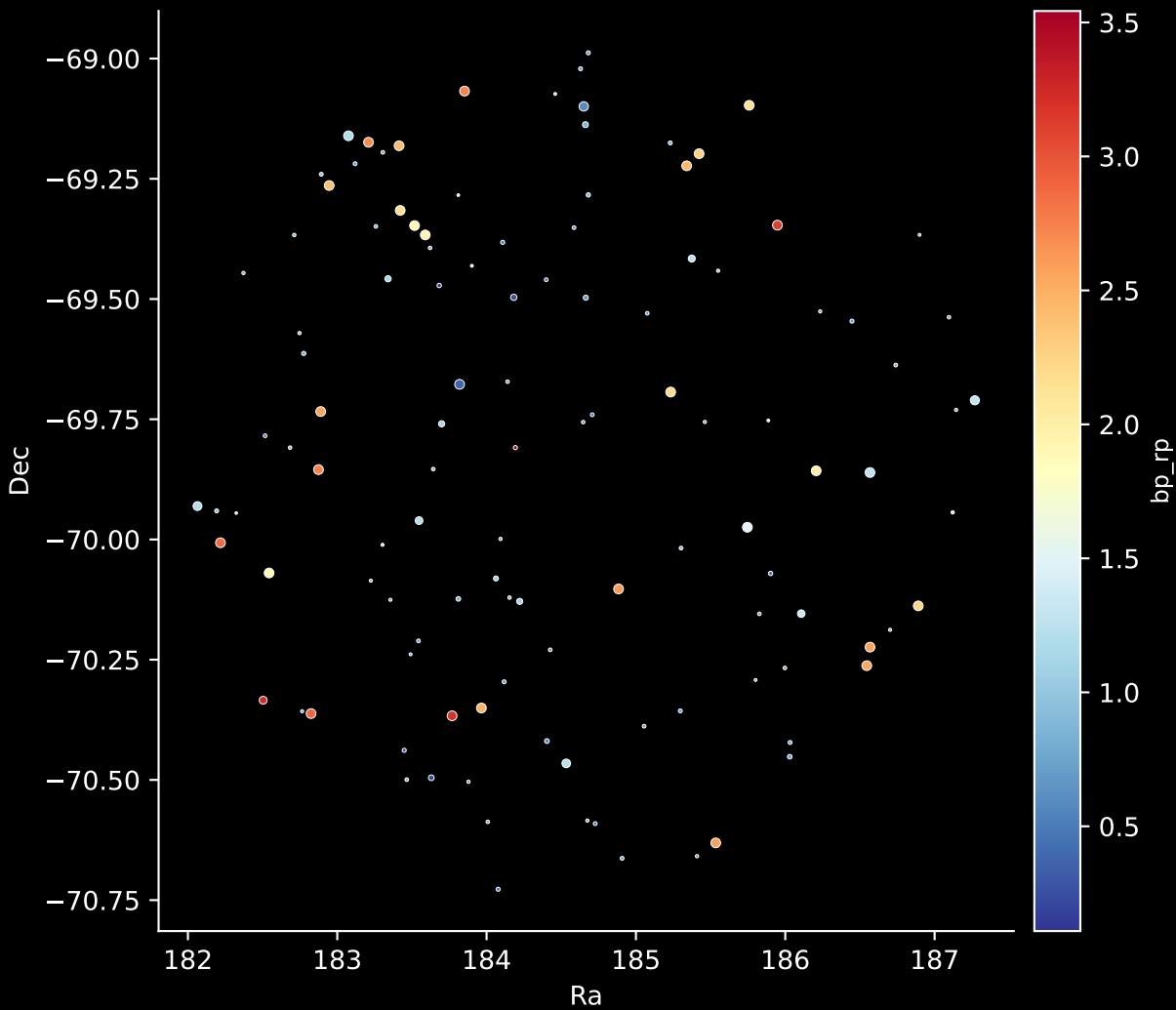
APOGEE DR17 Field: [280-32-O_TESS] Stars: 116
